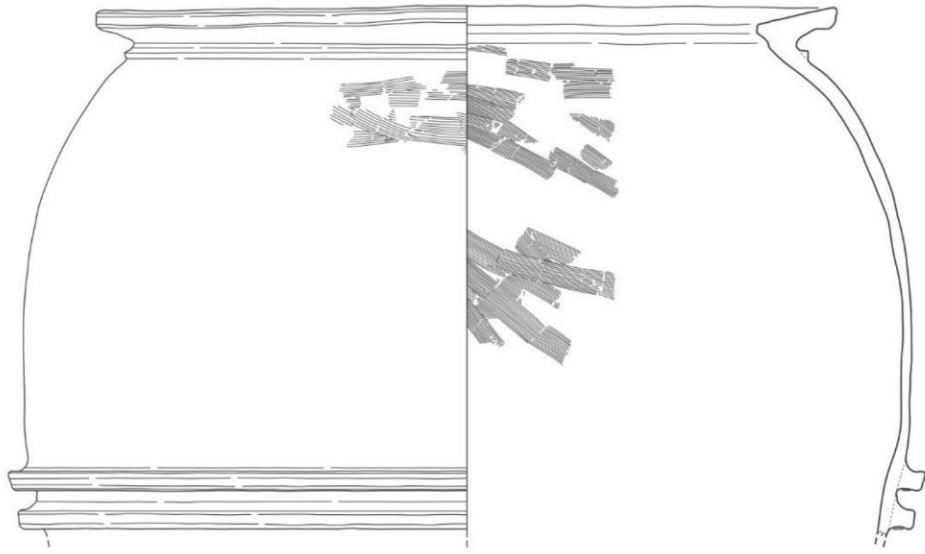
鉄戈が副葬された甕棺実測図（S = 3/20）
