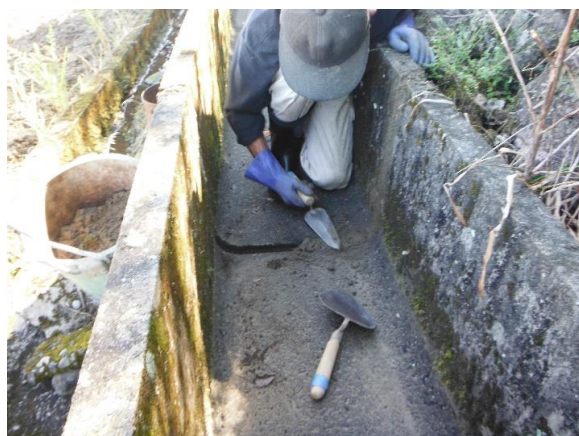
大殿墳 水路漏水箇所の補修 H29.5.4
