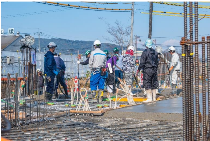
床コンクリートの打設後の様子→
