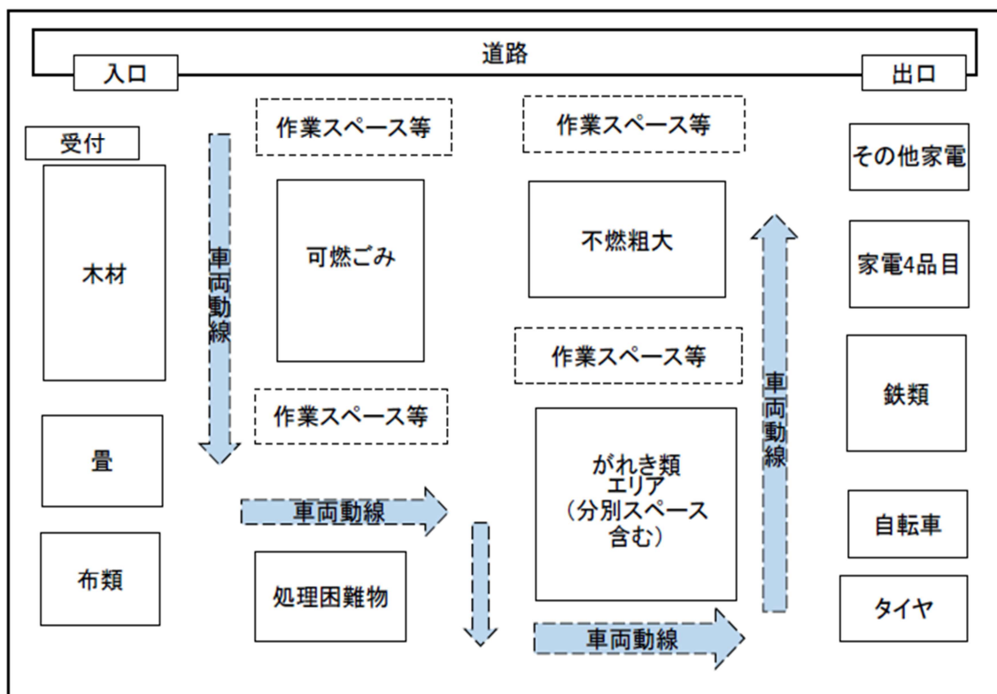
◇図表〔仮置き場のレイアウト（案）〕
