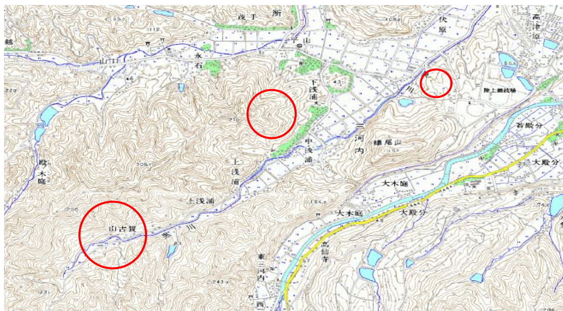
浅浦地区協定書取得測量調査の位置図
