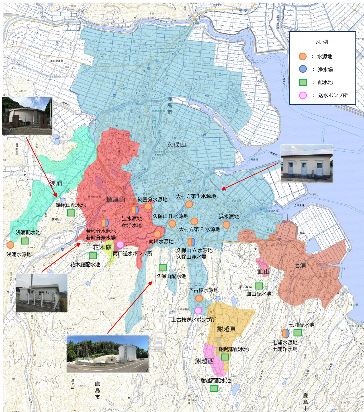
図2-3 給水区域と各施設位置図
