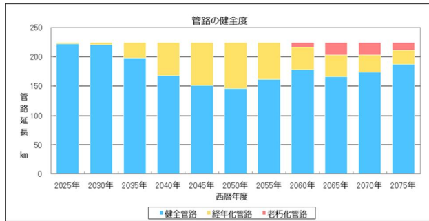
図4-3 管路の健全度の推移
