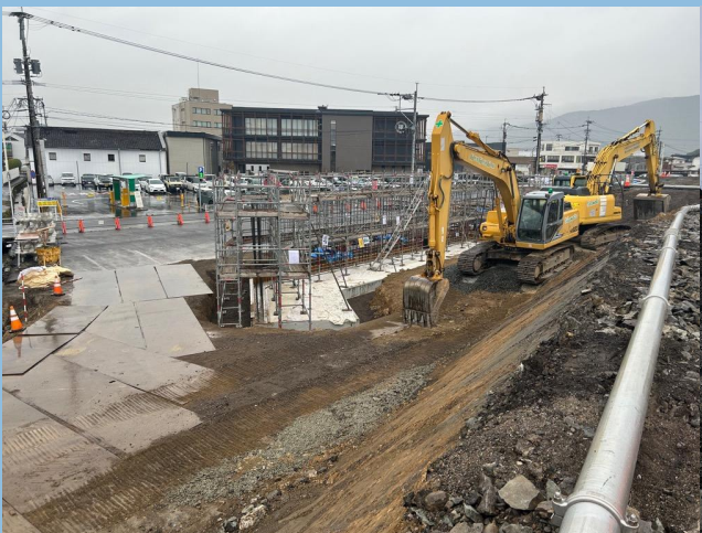
令和 8 年 2 月 新駅舎造成工事 擁壁・地盤改良
